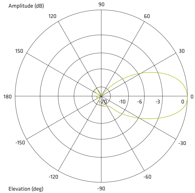
— Vertical-Plane: Copolar
